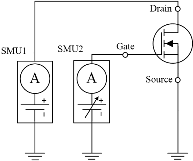
图2 双电压源扫描法测试电路
